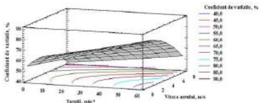
Figura 8. Uniformitatea distribuției semințelor și suprafața de răspuns a coeficientului de variație în raport cu turațiile cilindrului canelat și viteza aerului din tub la sistemul mecatronic
