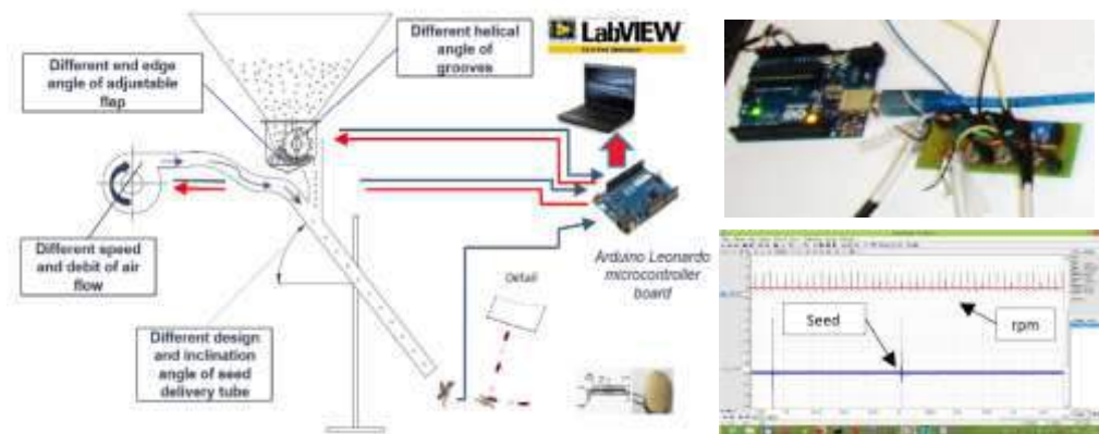
Figura 1. Schema principală de organizare a experiențelor pentru determinarea uniformității distribuției la sistemul mecatronic de distribuție a semințelor cu control digital semințelor.
