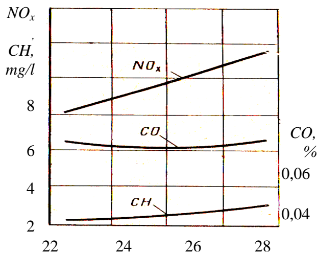
Fig. 2 Dependența toxicității gazelor de eșapament de unghiul avans la injecție \alpha_i
