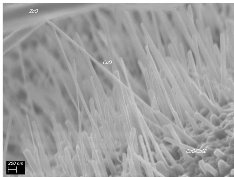
Figura 2. Imaginile SEM ale nanostructurilor de oxizi micști Zn-Cu la scara de 200 nm
