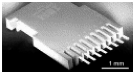
Рис. 1. Консольная матрица [1]
