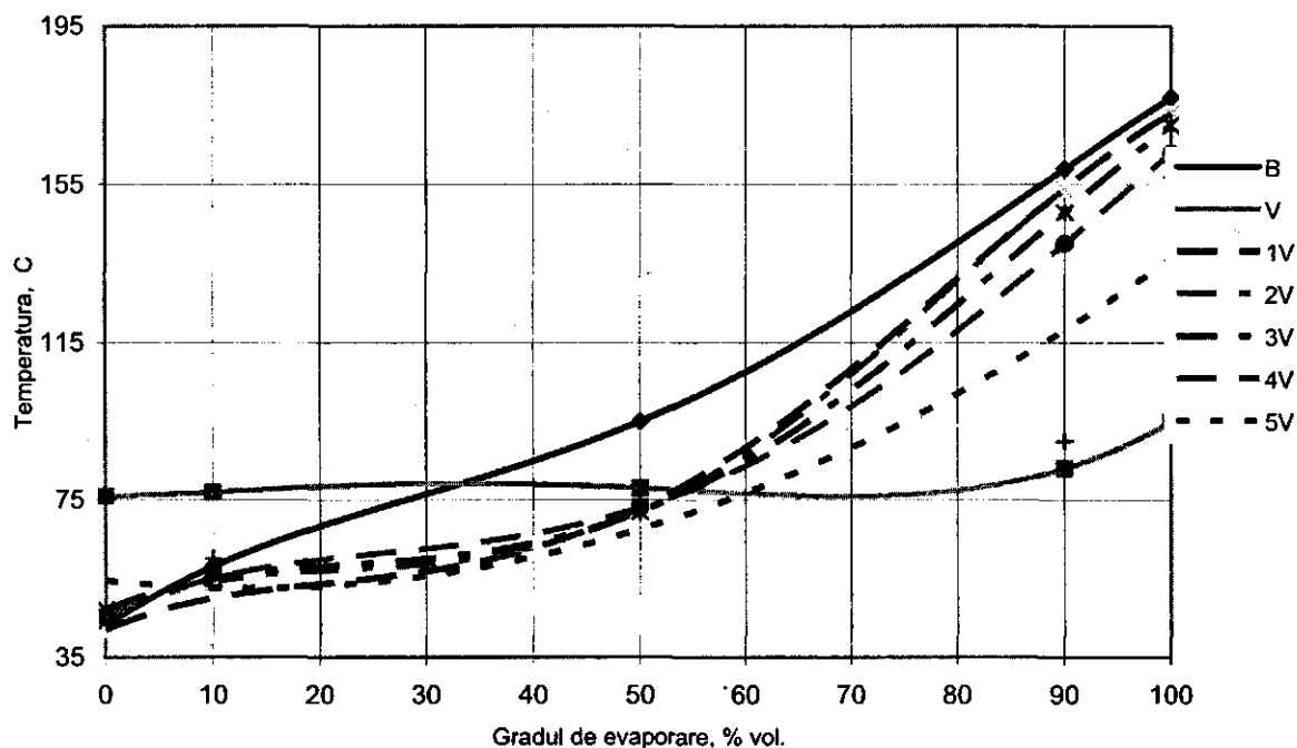
Fig.1. Modificarea componenței fracționale a combustibilului în baza benzinei A-92 (B) cu adaosul etanolului (V) din fracții frunte-coada (1V...5V- amestec cu concentrația etanolului V respectiv 10..50%)
