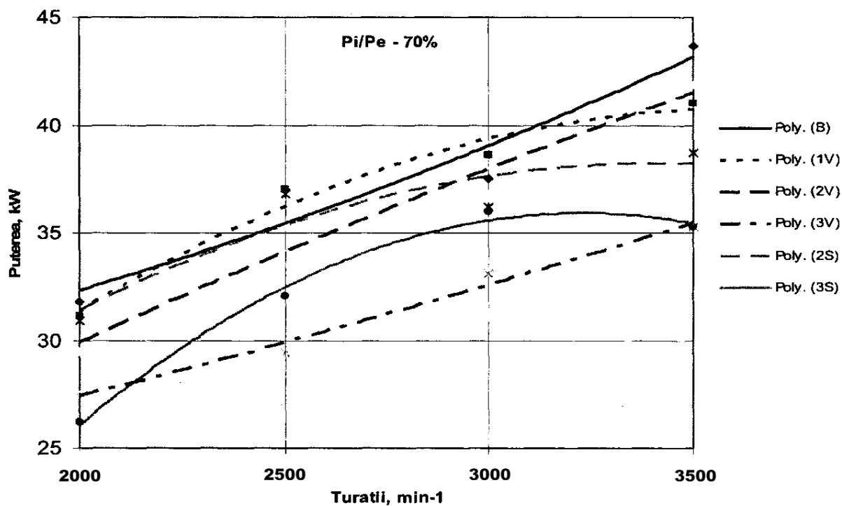
Fig. 6. Dependența puterii motorului de turațiile arborelui cotit ( P_i / P_e = \lambda - gradul de solicitare a MAI)
