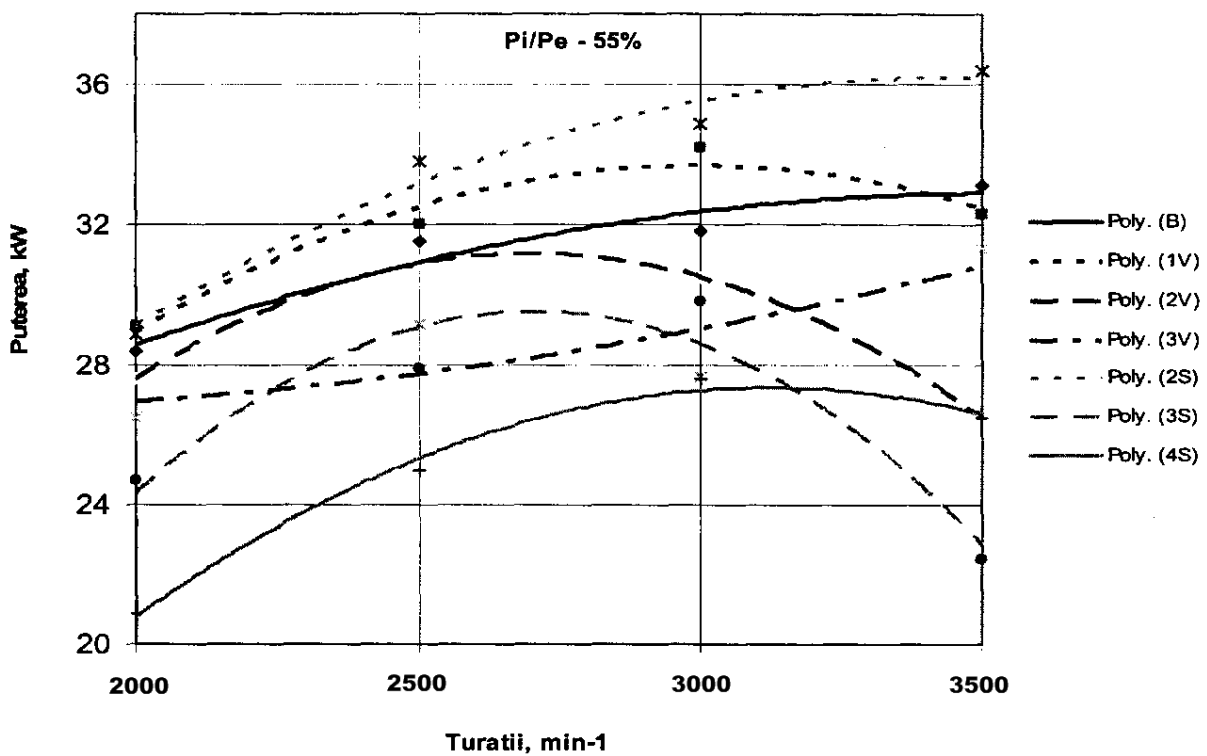
Fig. 5. Dependența puterii motorului de turațiile arborelui cotit ( P_i / P_e = \lambda - gradul de solicitare a MAI)
