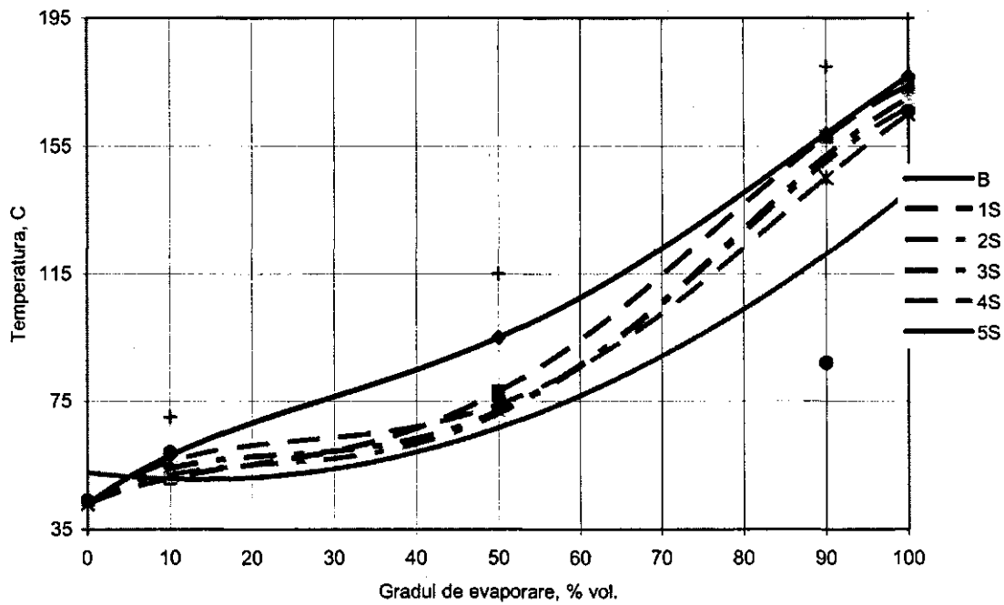
Fig.2. Modificarea componenței fracționale a combustibilului în baza benzinei A-92 (B) cu adaosul etanolului (S) din sorg zaharat (1S...5S - amestec cu concentrația etanolului S respectiv 10..50%)
