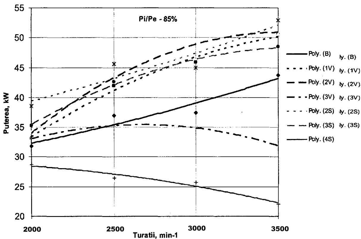
Fig. 7. Dependența puterii motorului de turațiile arborelui cotit ( P_i / P_e = \lambda - gradul de solicitare a MAI)
