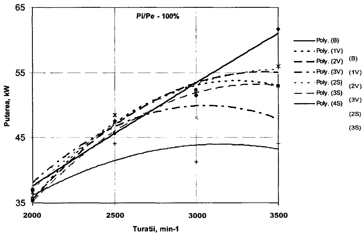
Fig. 8. Dependența puterii motorului de turațiile arborelui cotit ( P_i / P_e = \lambda - gradul de solicitare a MAI)
