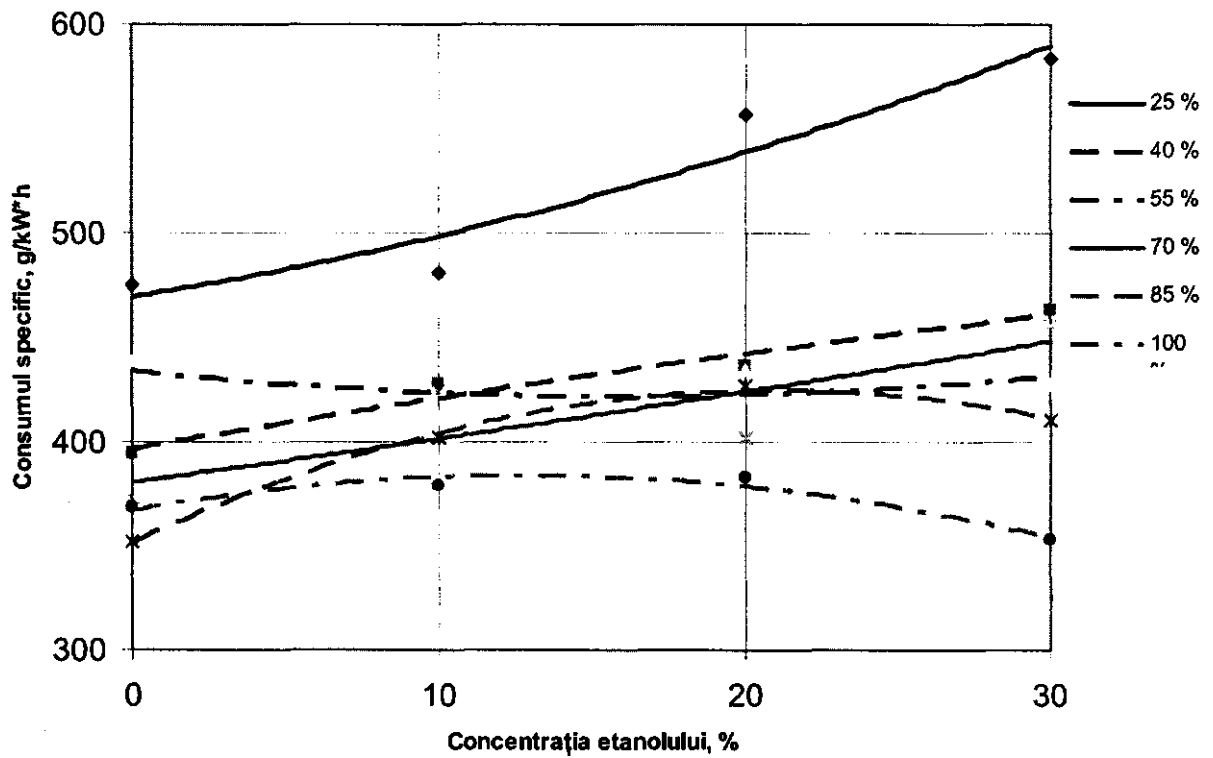
Fig. 13. Dependența consumului specific de concentrația etanolului obținut din fracții frunte-coadă din vinificație ( n=2000 \text{ min}^{-1} )
