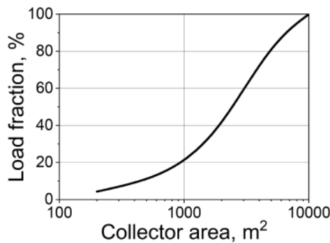
Рис. 3. Доля покрытия нагрузки в зависимости от площади солнечных коллекторов. Fig.3. Share of load coverage depending on the area of solar collectors.
