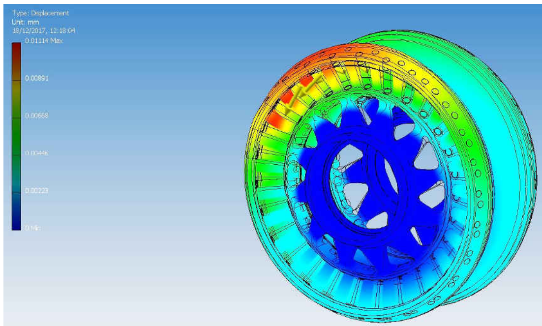
Fig. 2.13. Varianta constructivă a roții-satelit cu angrenare de tipul A^B_{CX-CV} ( Z_2 = 27 , Z_3 = 22 , \delta_{(1-2)} = \delta_{(3-4)} = 22,5^\circ , \beta_{(1-2)} = 3,5^\circ , \beta_{(3-4)} = 4,78^\circ , \theta = 3,5^\circ , R_m = 46 mm, r_2 = 2,9 mm, r_3 = 4,38 mm). Opțiunea 1.
