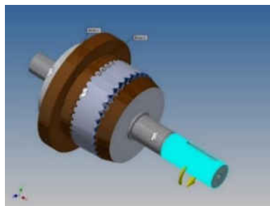
Fig. 4.29. Momentul de torsiune acceptat pentru transmisia precesională cu angrenare de tipul A^D_{CX-CV} ( Z_1 = 40 , Z_2 = 41 , Z_3 = 33 , Z_4 = 32 , \delta_{(1-2)} = \delta_{(3-4)} = 22,5^\circ , \beta_{(1-2)} = 3,2^\circ , \beta_{(3-4)} = 3,5^\circ , \theta = 3,5^\circ , R_m = 19 mm, i = -164 )
