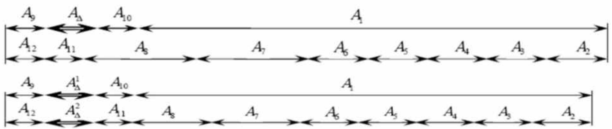
Fig. 3.8. Lanțul dimensional al reductorului precasional de tipul A B cx-cv cu două elemente funcționale
