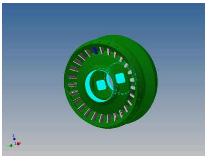
Fig. A2.14. Varianta constructivă de bază a roții-satelit cu angrenare de tip A B CX-CV ( Z_2 = 27, Z_3 = 22, \delta_{(1-2)} = \delta_{(3-4)} = 22,5^\circ, \beta_{(1-2)} = 3,5^\circ, \beta_{(3-4)} = 4,78^\circ, \theta = 3,5^\circ, R_m = 46 \text{ mm}, r_2 = 2,9 \text{ mm}, r_3 = 4,38 \text{ mm} ).
