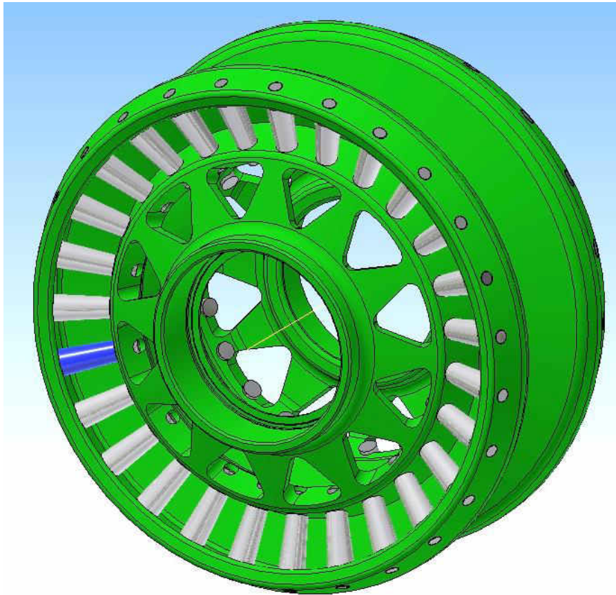
Fig. 2.12. Varianta constructivă a roții-satelit cu angrenare de tipul A^B_{CX-CV} ( Z_2 = 27 , Z_3 = 22 , \delta_{(1-2)} = \delta_{(3-4)} = 22,5^\circ , \beta_{(1-2)} = 3,5^\circ , \beta_{(3-4)} = 4,78^\circ , \theta = 3,5^\circ , R_m = 46 mm, r_2 = 2,9 mm, r_3 = 4,38 mm). Opțiunea 1
