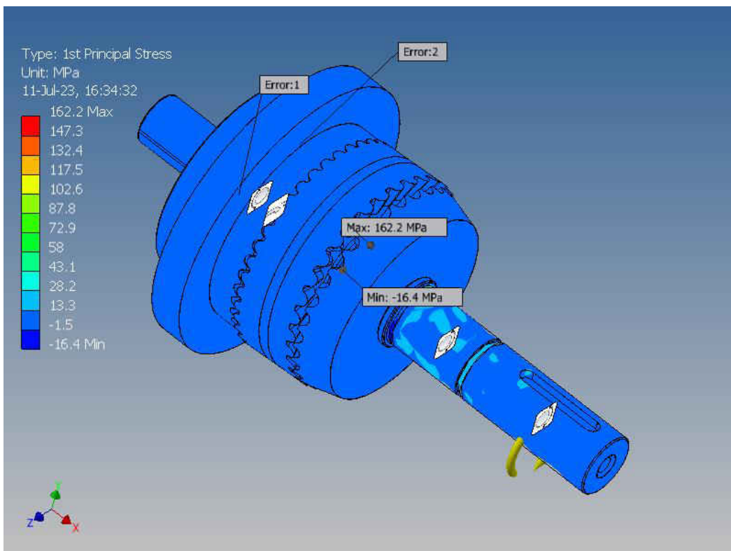
Fig. A2.3. 1-a tensiune de bază a transmisiei precesionale cu angrenare de tip A^D_{CX-CV} ( Z_1 = 40 , Z_2 = 41 , Z_3 = 33 , Z_4 = 32 , \delta_{(1-2)} = \delta_{(3-4)} = 22,5^\circ , \beta_{(1-2)} = 3,2^\circ , \beta_{(3-4)} = 3,5^\circ , \theta = 3,5^\circ , R_m = 19 mm, i = -164 ), MPa
