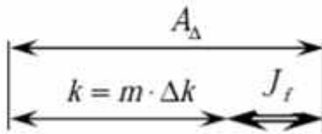
Fig. 3.3. Lanțul dimensional al compensatorului transmisie planetară precesională pentru asigurarea jocului funcțional
