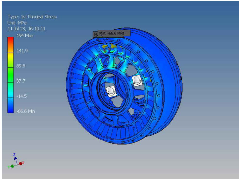
Fig. A2.52. Opțiunea constructivă 3 a roții-satelit cu angrenare de tip A^B_{CX-CV} ( Z_2 = 27 , Z_3 = 22 , \delta_{(1-2)} = \delta_{(3-4)} = 22,5^\circ , \beta_{(1-2)} = 3,5^\circ , \beta_{(3-4)} = 4,78^\circ , \theta = 3,5^\circ , R_m = 46 mm, r_2 = 2,9 mm, r_3 = 4,38 mm). 1-a tensiune principală, MPa
