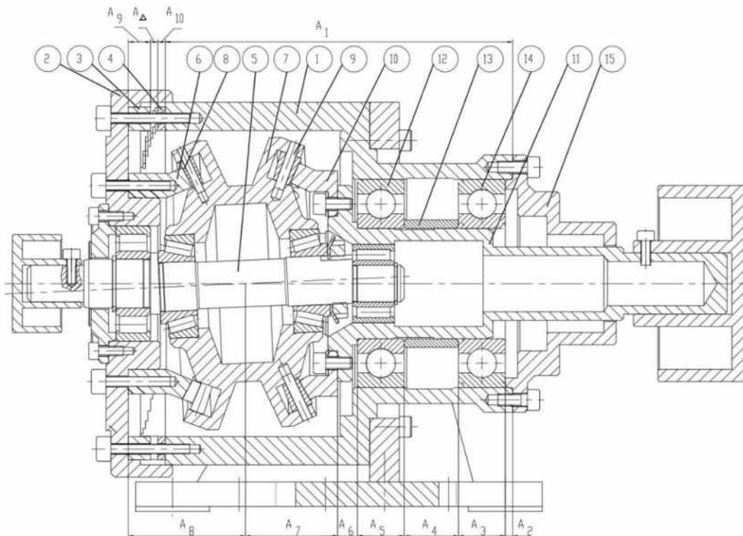
Fig. 3.4. Secțiunea unui reductor precusional cu tipul de angrenaj A^B cx-cv cu un element compensator
