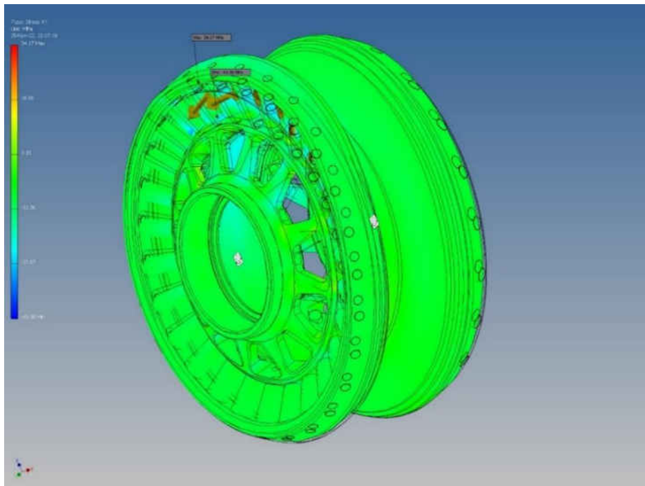
Fig. 4.14. Varianta constructivă optimizată a roții-satelit cu angrenare de tipul A^B_{CX-CV} ( Z_2 = 27 , Z_3 = 22 , \delta_{(1-2)} = \delta_{(3-4)} = 22,5^\circ , \beta_{(1-2)} = 3,5^\circ , \beta_{(3-4)} = 4,78^\circ , \theta = 3,5^\circ , R_m = 46 mm, r_2 = 2,9 mm, r_3 = 4,38 mm).
