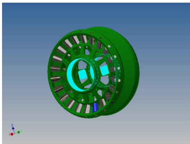
Fig. A2.50. Opțiunea constructivă 3 a roții-satelit cu angrenare de tip A B CX-CV ( Z_2 = 27, Z_3 = 22, \delta_{(1-2)} = \delta_{(3-4)} = 22,5^\circ, \beta_{(1-2)} = 3,5^\circ, \beta_{(3-4)} = 4,78^\circ, \theta = 3,5^\circ, R_m = 46 \text{ mm}, r_2 = 2,9 \text{ mm}, r_3 = 4,38 \text{ mm} ). Elemente de fixare
