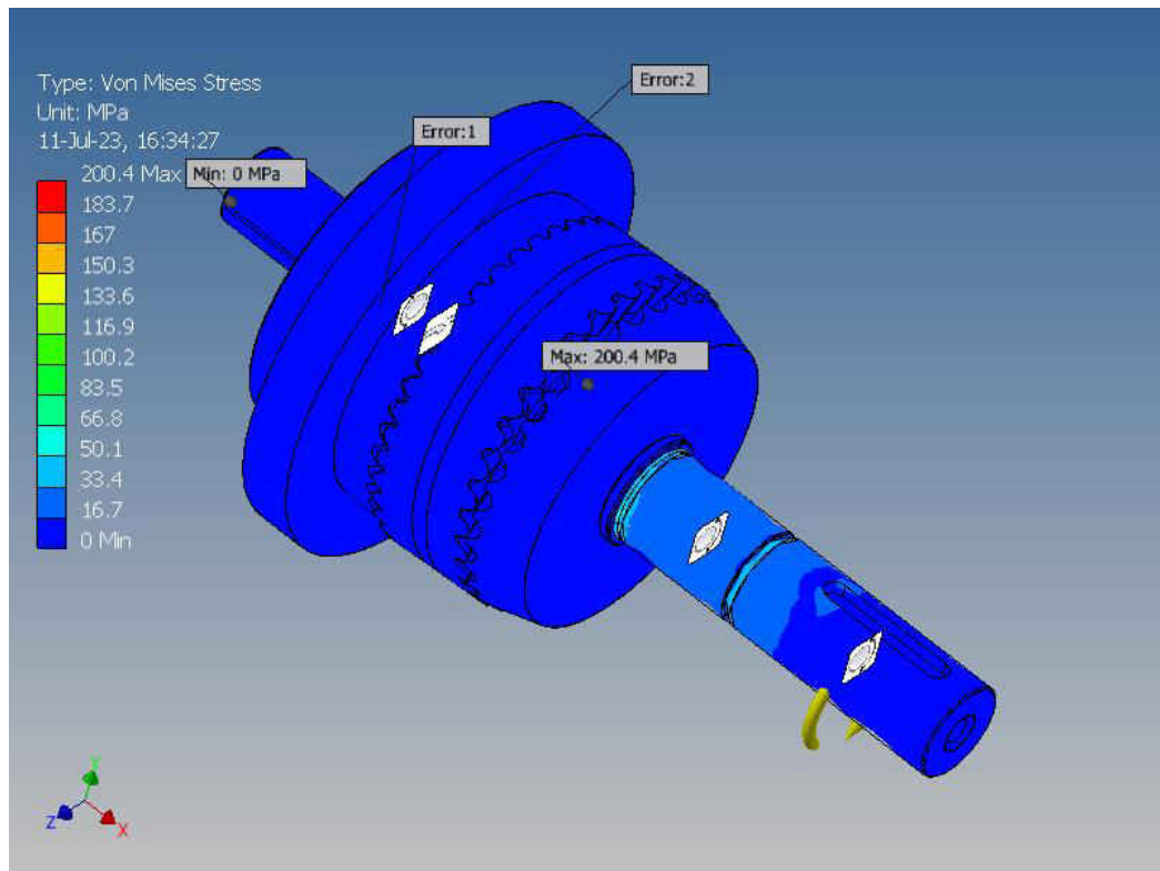
Fig. A2.2. Tensiune echivalentă a transmisiei precesionale cu angrenare de tip A^D_{CX-CV} ( Z_1 = 40 , Z_2 = 41 , Z_3 = 33 , Z_4 = 32 , \delta_{(1-2)} = \delta_{(3-4)} = 22,5^\circ , \beta_{(1-2)} = 3,2^\circ , \beta_{(3-4)} = 3,5^\circ , \theta = 3,5^\circ , R_m = 19 mm, i = -164 ) de Von Mises, MPa
