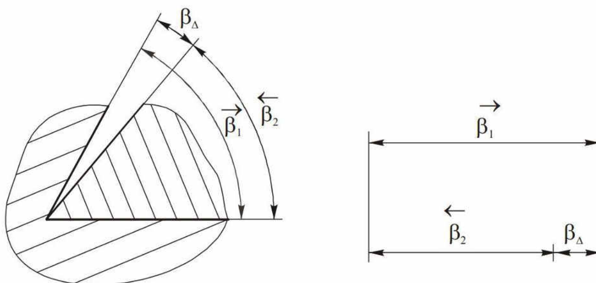
Fig. 1.5. Lanț dimensional unghiular
