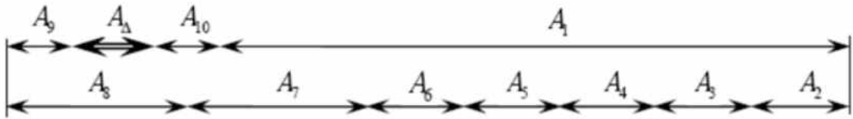
Fig. 3.5. Lanțul dimensional al reductorului precesional de tipul A B ex-cv cu un element compensator
