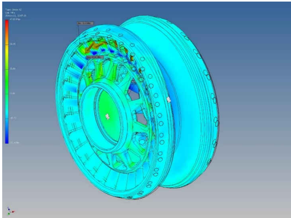
Fig. 4.15. Varianta constructivă optimizată a roții-satelit cu angrenare de tipul A^B_{CX-CV} ( Z_2 = 27 , Z_3 = 22 , \delta_{(1-2)} = \delta_{(3-4)} = 22,5^\circ , \beta_{(1-2)} = 3,5^\circ , \beta_{(3-4)} = 4,78^\circ , \theta = 3,5^\circ , R_m = 46 mm, r_2 = 2,9 mm, r_3 = 4,38 mm).
