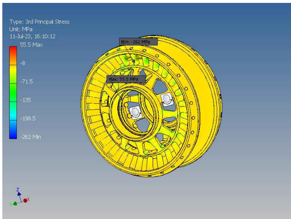
Fig. A2.53. Opțiunea constructivă 3 a roții-satelit cu angrenare de tip A^B_{CX-CV} ( Z_2 = 27 , Z_3 = 22 , \delta_{(1-2)} = \delta_{(3-4)} = 22,5^\circ , \beta_{(1-2)} = 3,5^\circ , \beta_{(3-4)} = 4,78^\circ , \theta = 3,5^\circ , R_m = 46 mm, r_2 = 2,9 mm, r_3 = 4,38 mm). A 3-ea tensiune principală, MPa
