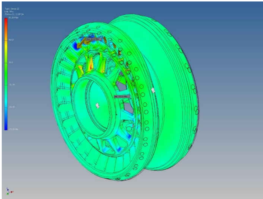
Fig. 4.18. Varianta constructivă optimizată a roții-satelit cu angrenare de tipul A B CX-CV ( Z_2 = 27 , Z_3 = 22 , \delta_{(1-2)} = \delta_{(3-4)} = 22,5^\circ , \beta_{(1-2)} = 3,5^\circ , \beta_{(3-4)} = 4,78^\circ , \theta = 3,5^\circ , R_m = 46 mm, r_2 = 2,9 mm, r_3 = 4,38 mm).
