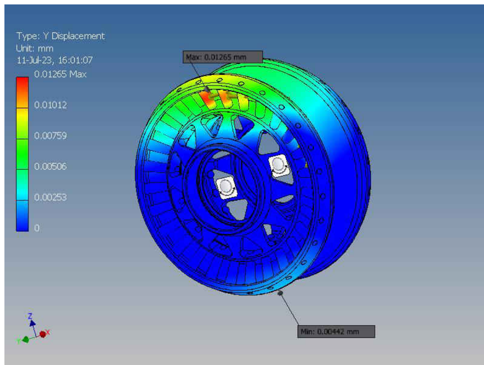
Fig. A2.36. Opțiunea constructivă 1 a roții-satelit cu angrenare de tip A^B_{CX-CV} ( Z_2 = 27, Z_3 = 22, \delta_{(1-2)} = \delta_{(3-4)} = 22,5^\circ, \beta_{(1-2)} = 3,5^\circ, \beta_{(3-4)} = 4,78^\circ, \theta = 3,5^\circ, R_m = 46 \text{ mm}, r_2 = 2,9 \text{ mm}, r_3 = 4,38 \text{ mm} ).
