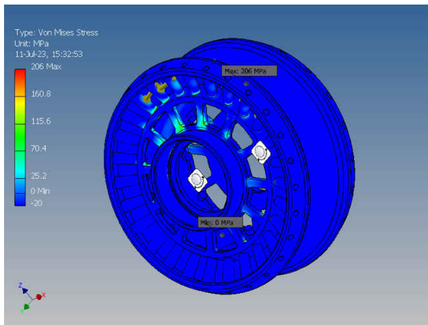
Fig. A2.63. Opțiunea constructivă 4 a roții-satelit cu angrenare de tip A^B_{CX-CV} ( Z_2 = 27 , Z_3 = 22 , \delta_{(1-2)} = \delta_{(3-4)} = 22,5^\circ , \beta_{(1-2)} = 3,5^\circ , \beta_{(3-4)} = 4,78^\circ , \theta = 3,5^\circ , R_m = 46 mm, r_2 = 2,9 mm, r_3 = 4,38 mm).
