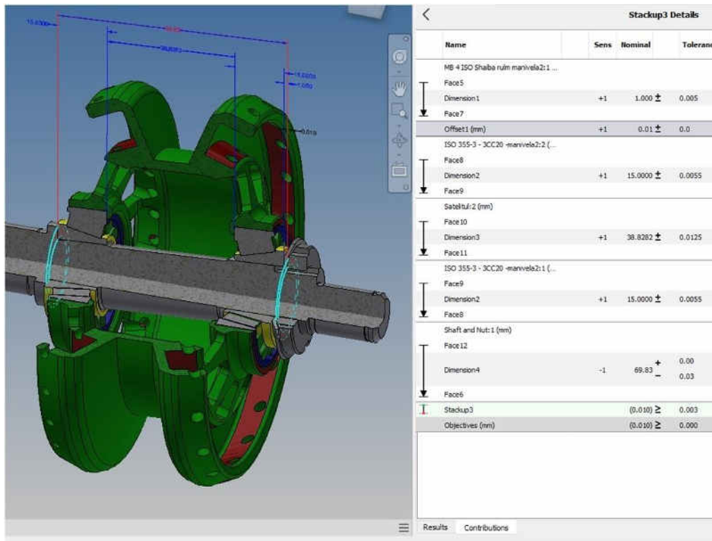
Fig. 3.34. Influența valorii toleranțelor calculate (în raport procentual) ale elementelor transmisiei precesionale cu angrenare de tipul A^B_{CX-CV} ( Z_2 = 27 , Z_3 = 22 , \delta_{(1-2)} = \delta_{(3-4)} = 22,5^\circ , \beta_{(1-2)} = 3,5^\circ , \beta_{(3-4)} = 4,78^\circ , \theta = 3,5^\circ , R_m = 46 mm, r_2 = 2,9 mm, r_3 = 4,38 mm)
