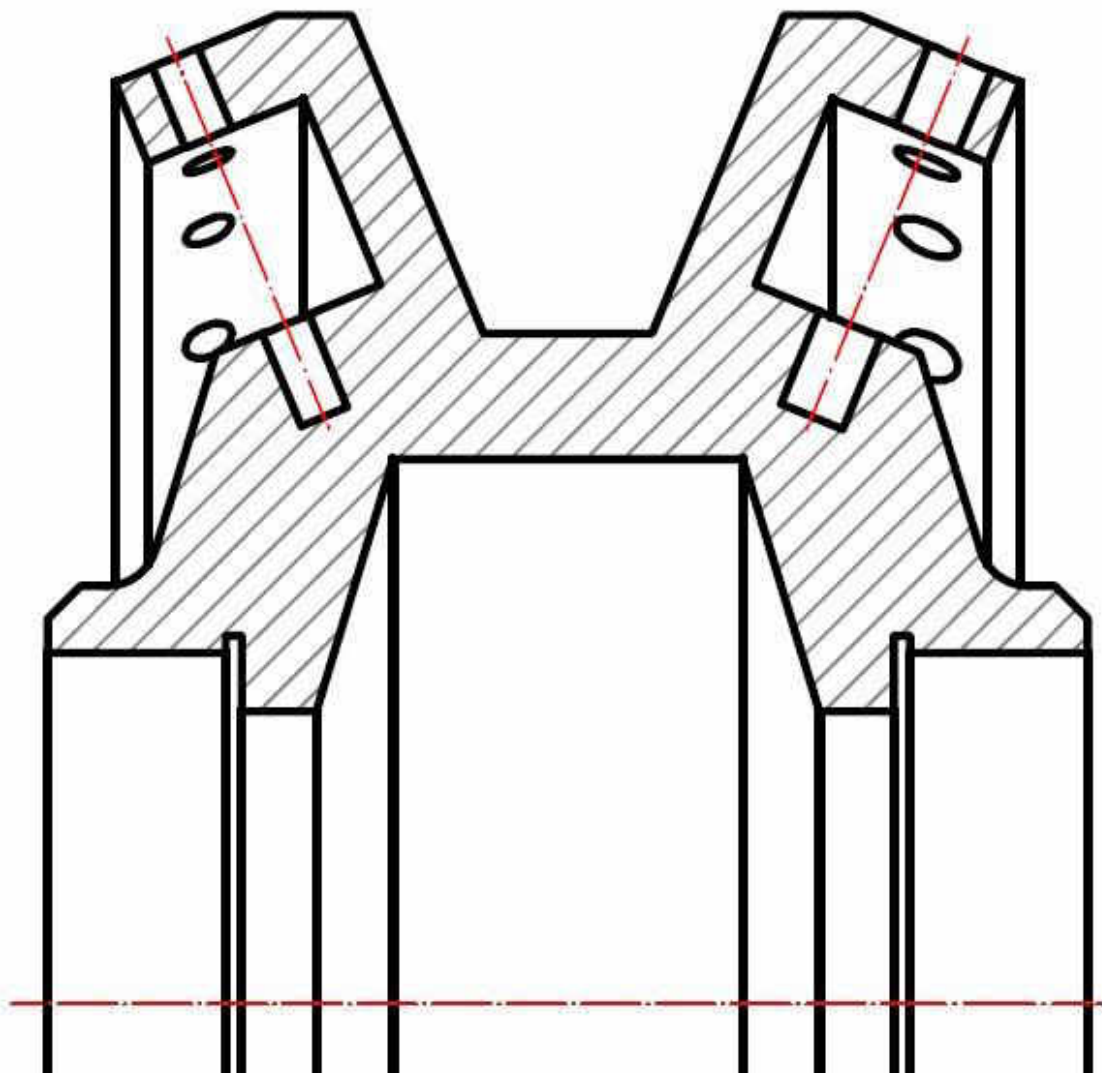
Fig. 2.11. Varianta constructivă de bază a roții-satelit cu angrenare de tipul A^B_{CX-CV} ( Z_2 = 27 , Z_3 = 22 , \delta_{(1-2)} = \delta_{(3-4)} = 22,5^\circ , \beta_{(1-2)} = 3,5^\circ , \beta_{(3-4)} = 4,78^\circ , \theta = 3,5^\circ , R_m = 46 mm, r_2 = 2,9 mm, r_3 = 4,38 mm).
