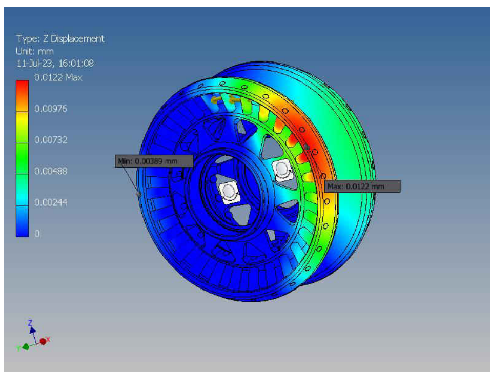
Fig. A2.37. Opțiunea constructivă 1 a roții-satelit cu angrenare de tip A^B_{CX-CV} ( Z_2 = 27, Z_3 = 22, \delta_{(1-2)} = \delta_{(3-4)} = 22,5^\circ, \beta_{(1-2)} = 3,5^\circ, \beta_{(3-4)} = 4,78^\circ, \theta = 3,5^\circ, R_m = 46 \text{ mm}, r_2 = 2,9 \text{ mm}, r_3 = 4,38 \text{ mm} ).
