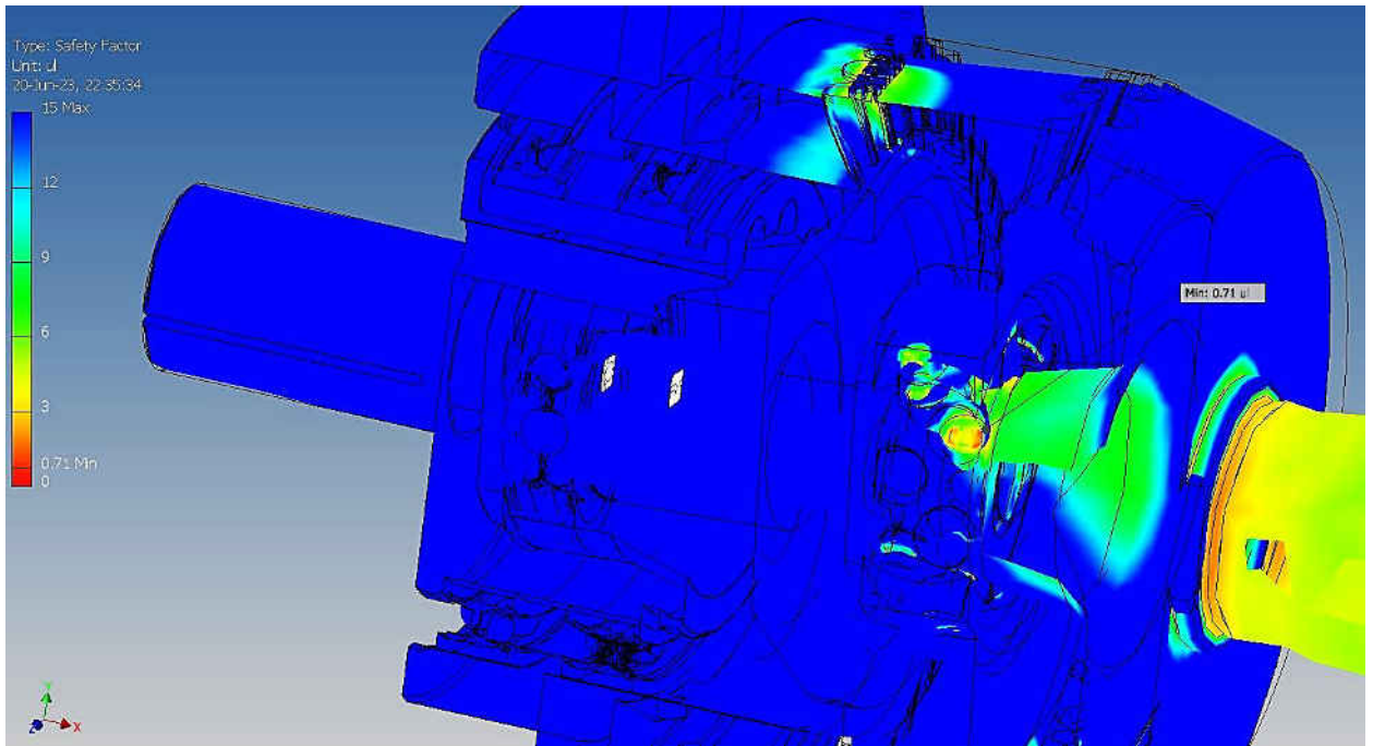
Fig. 4.36. Valoarea coeficientului de siguranță a rulmentului cu autoaşezare. Momentul de torsiune de 15 Nm
