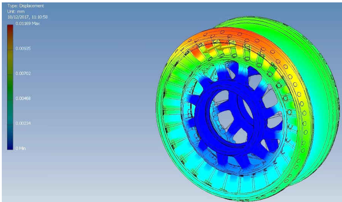
Fig. 2.17. Varianta constructivă a roții-satelit cu angrenare de tipul A^B_{CX-CV} ( Z_2 = 27 , Z_3 = 22 , \delta_{(1-2)} = \delta_{(3-4)} = 22,5^\circ , \beta_{(1-2)} = 3,5^\circ , \beta_{(3-4)} = 4,78^\circ , \theta = 3,5^\circ , R_m = 46 mm, r_2 = 2,9 mm, r_3 = 4,38 mm). Opțiunea 3.
