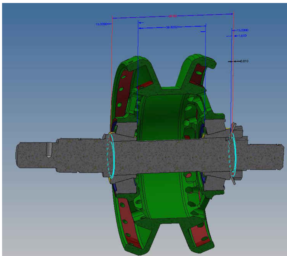
Fig. 3.35. Dimensiunea elementelor transmisiei precesonale cu angrenare de tipul A^B_{CX-CV} ( Z_2 = 27 , Z_3 = 22 , \delta(1-2) = \delta(3-4) = 22,5^\circ , \beta(1-2) = 3,5^\circ , \beta(3-4) = 4,78^\circ , \Theta = 3,5^\circ , R_m = 46 mm, r_2 = 2,9 mm, r_3 = 4,38 mm)
