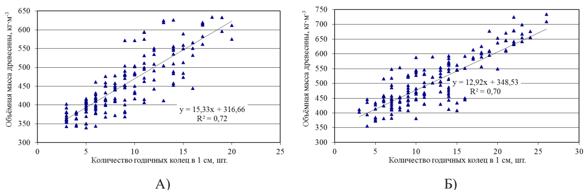
Рисунок 2. Зависимость между объёмной массой древесины и числом годичных колец в 1 см: А – пробная площадь №1 и Б – пробная площадь №2
