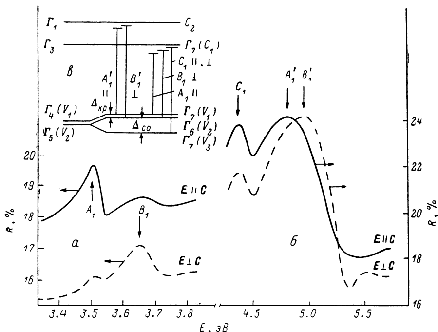
Спектры отражения кристаллов \text{CuAlS}_2 при 77 К ( a , б ) и структура энергетических зон \text{CuAlS}_2 в точке K=0 зоны Бриллюэна ( в ).
